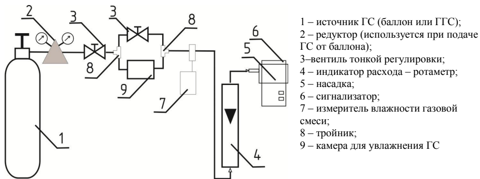
Рисунок 1 – Рекомендуемая схема подачи ГС на вход сигнализатора при проведении поверки
